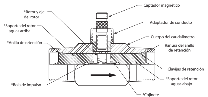
Figura 1: Componentes del caudalímetro
