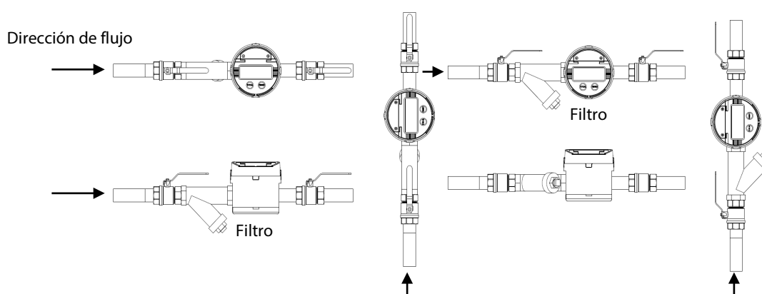
Ilustración 1: Instalación del medidor
