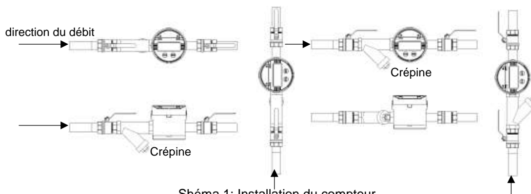
Shéma 1: Installation du compteur
